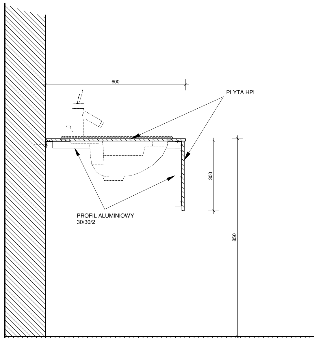
PRZEKROJ A - A
